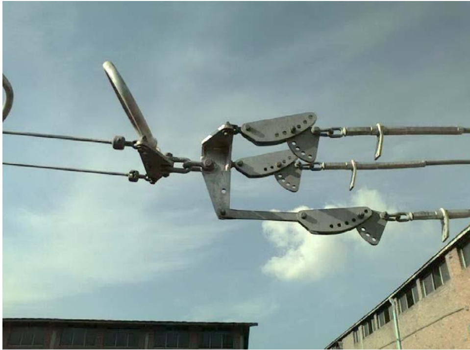
( استفاده از شکل ۳۸ , Socket Clevis , Yoke Plate , Arcing Rocket , Shackle , Sag Adjuster , Dead End Clamp , Extension Link
