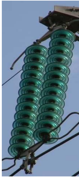
شکل ۲۹) زنجیره مفره آویزی
