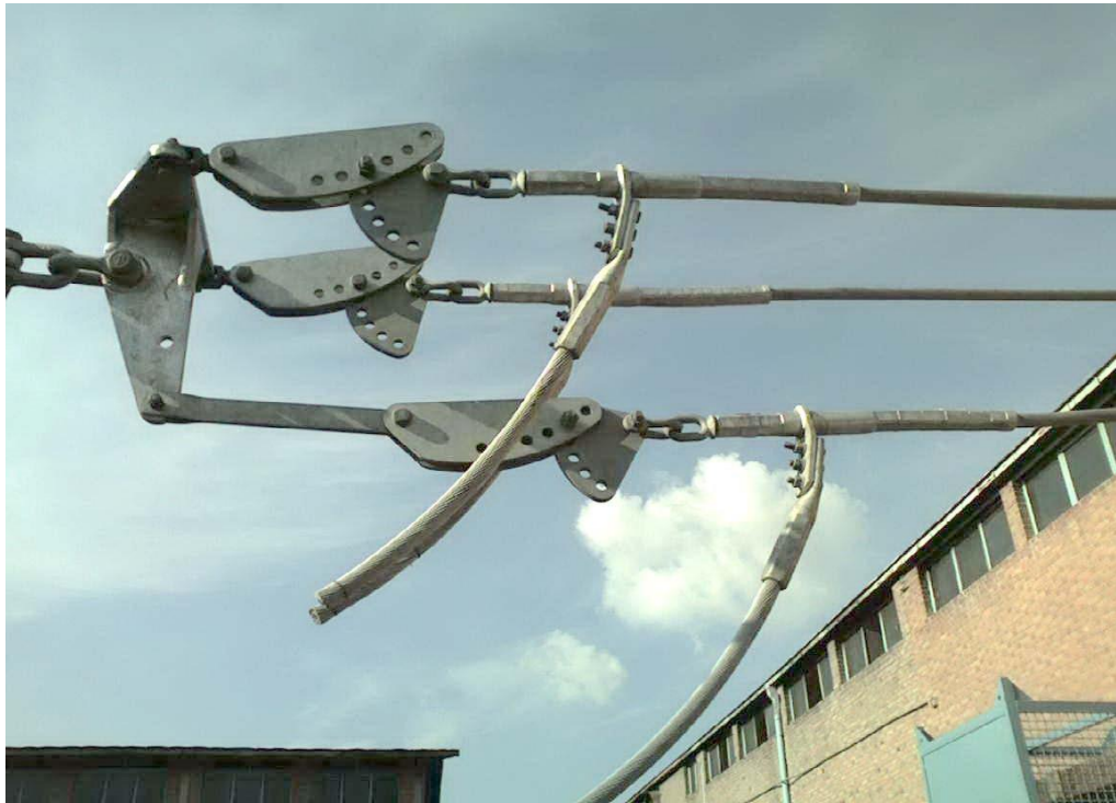
( استفاده از شکل ۳۹ ، Yoke Plate ، Socket Clevis ، Extension Link ، Shackle ، Sag Adjuster ، Dead End Clamp
