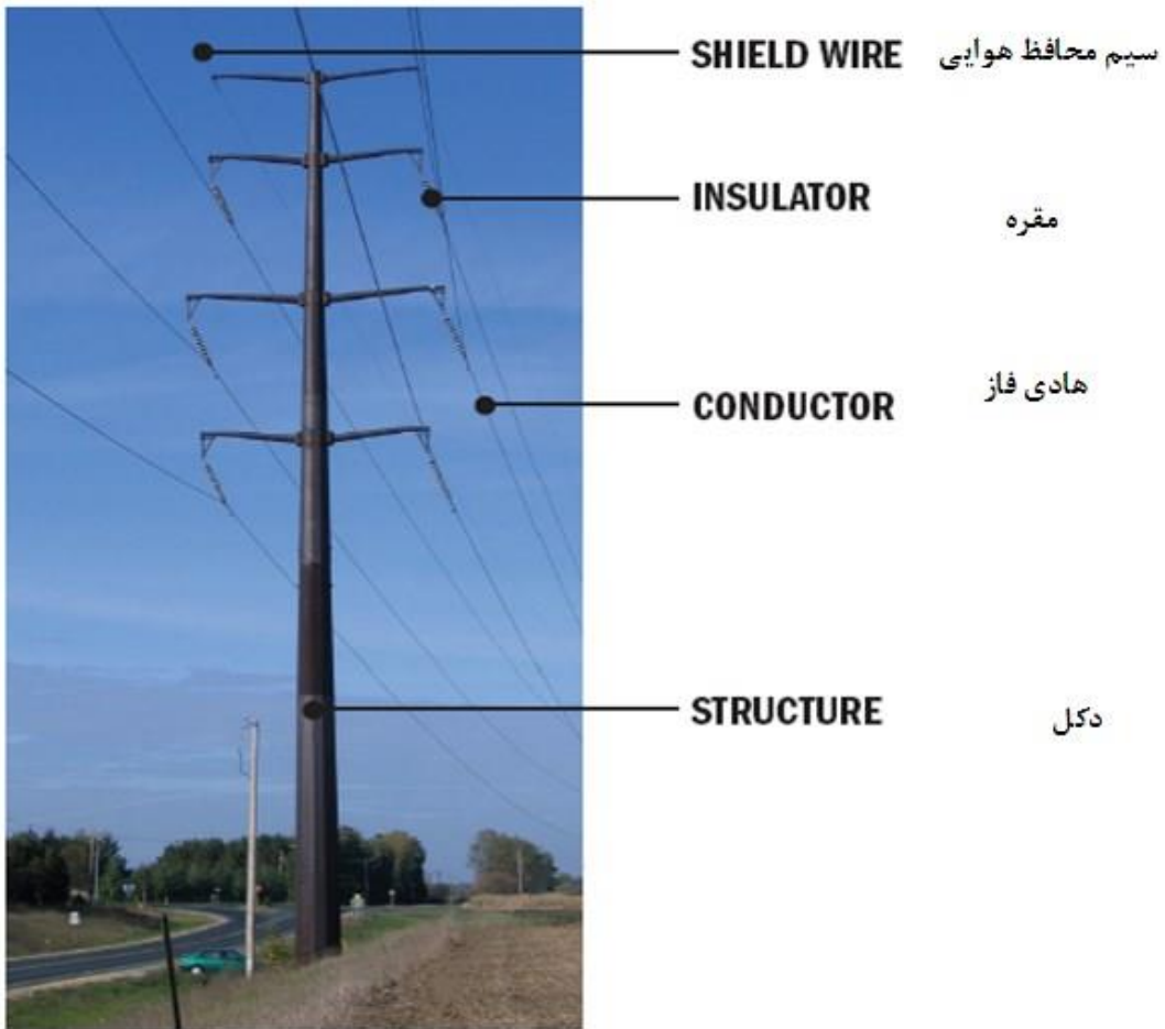
شكل ٢) اجزاء خط انتقال نيرو
