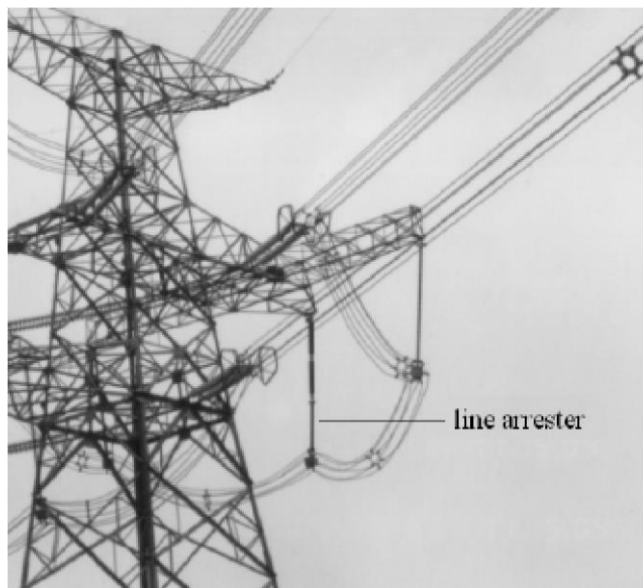
شکل ۴۶) نمایی از برگزیر خط بر روی دکل
