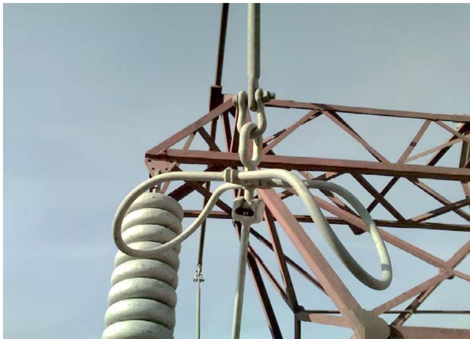
( استفاده از شکل ۳۷) Shackle , Ball Oval Eye , Arcing Rocket
